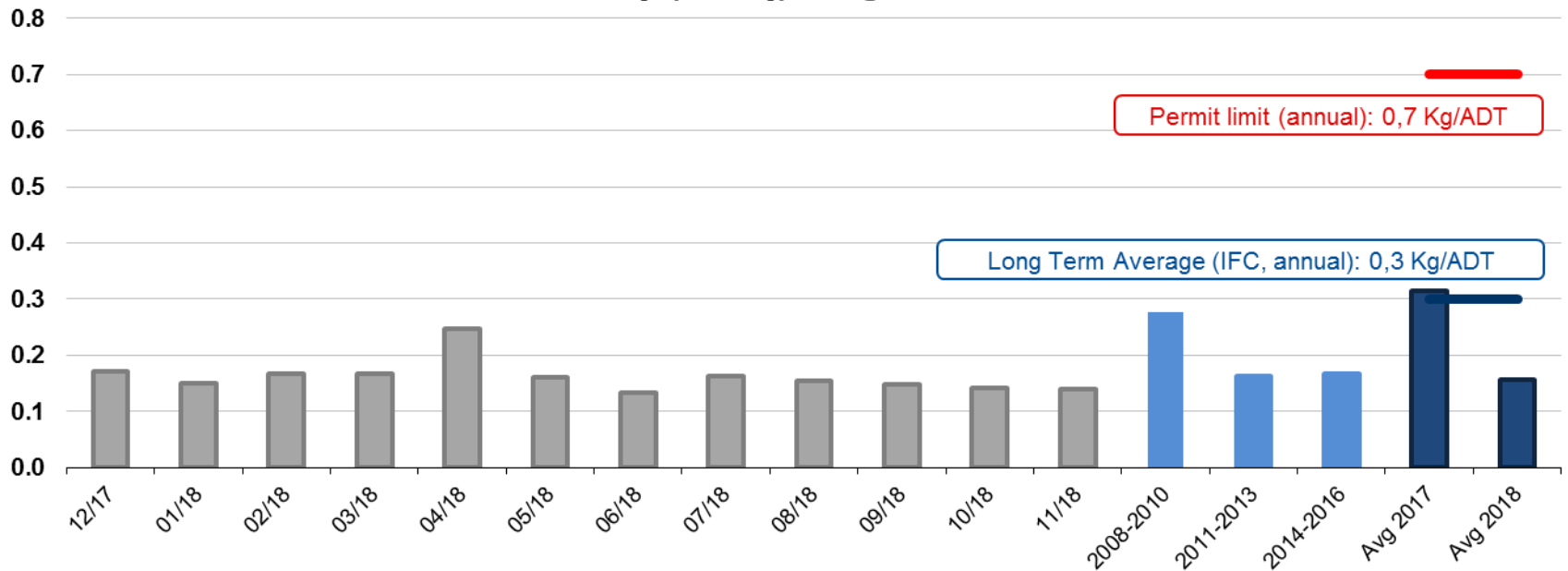
BOD 5 (DBO 5 ) - Kg/ADT
