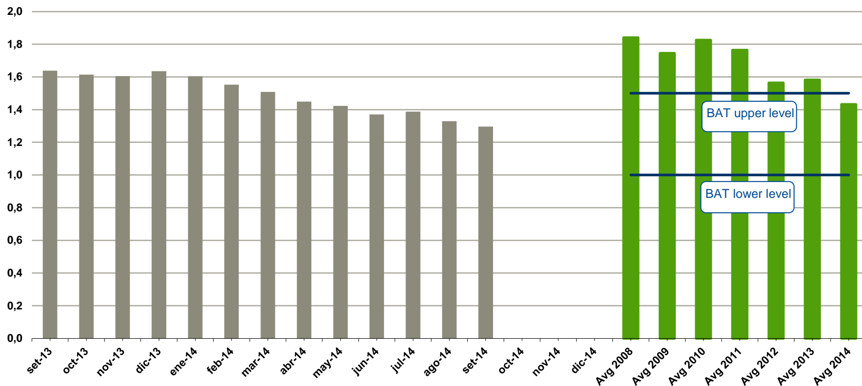
NOx - Kg/ADT
